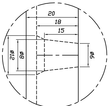
Hole Qty: 156 Det.A
